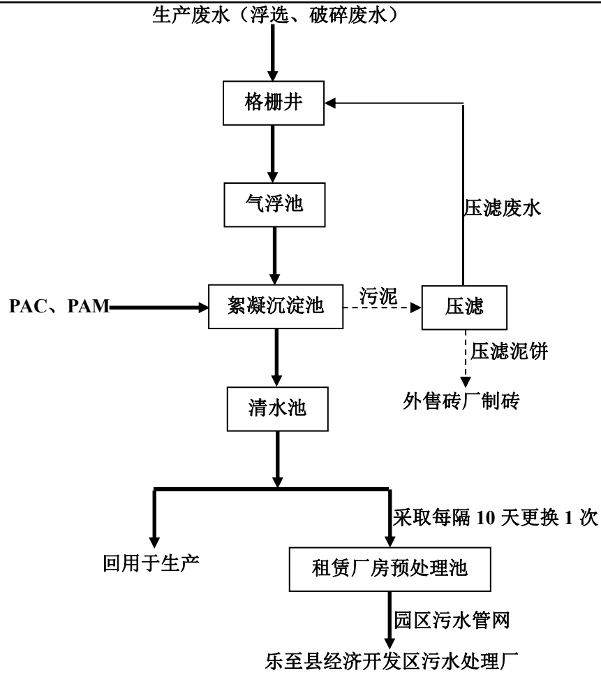
图 4-1 项目生产废水处理工艺图
